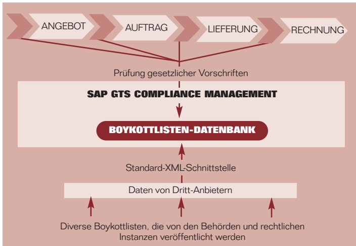
Abbildung 1: Boykottlisten-Prüfung
